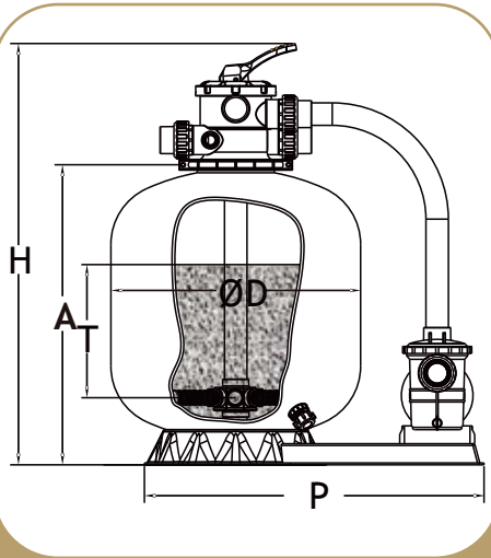
EB350~EB700
